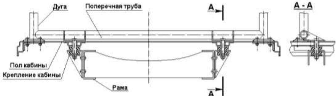
Рис. 7. Опоры главной дуги на грузовой платформе.
