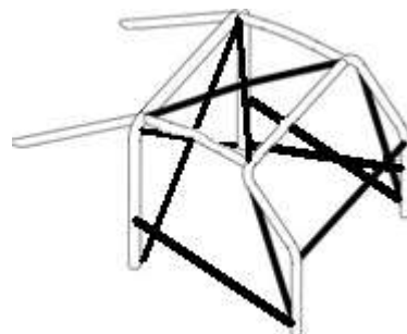
Рис. 1В (Рекомендуемая схема).
