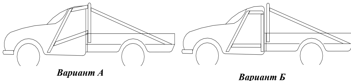
Рис. 11. Варианты каркаса безопасности с элементами внутри кабины.
