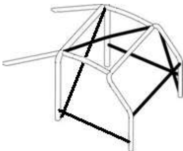
Рис. 1А (Минимально необходимая схема).
